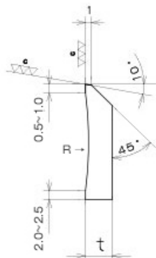
A-A矢視
